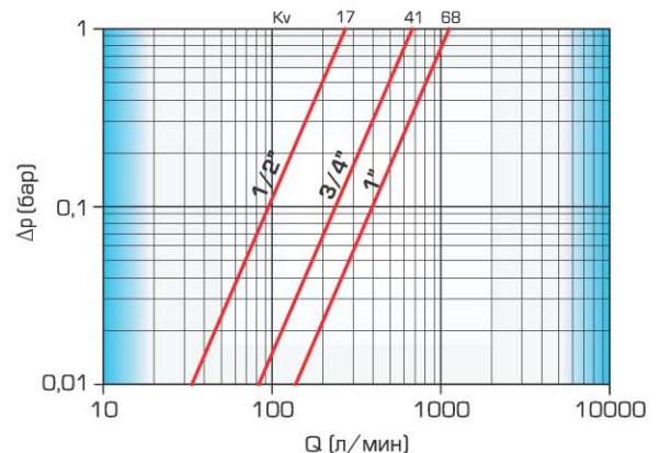
Диаграмма потока / падения давления Flow / pressure drop diagram
