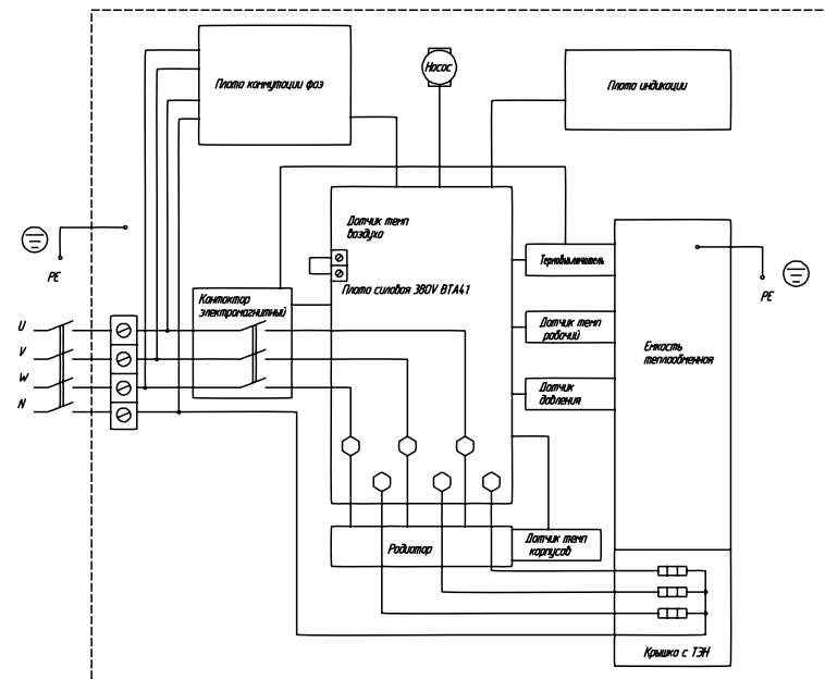
Рисунок 7 Схема подключения Wargos-RX-75-18 (380В)
