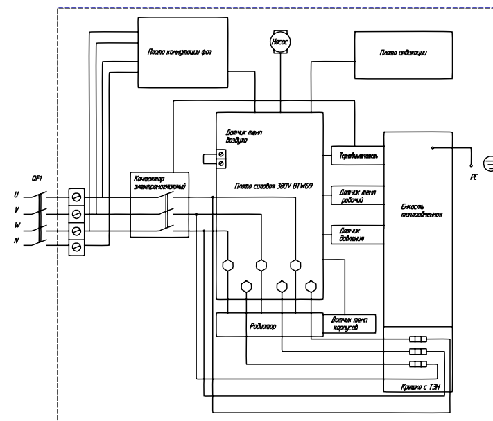
Рисунок 8 Схема подключения Wargos-RX-21-30
